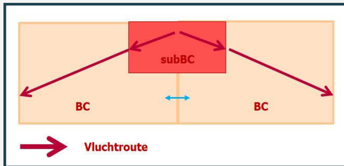
Figuur c: Ontvluchtingssystematiek bij 2 onafhankelijke toegangen vanaf het subBC en vervolgens 2 vluchtroutes (bron: Ministerie BZK)
