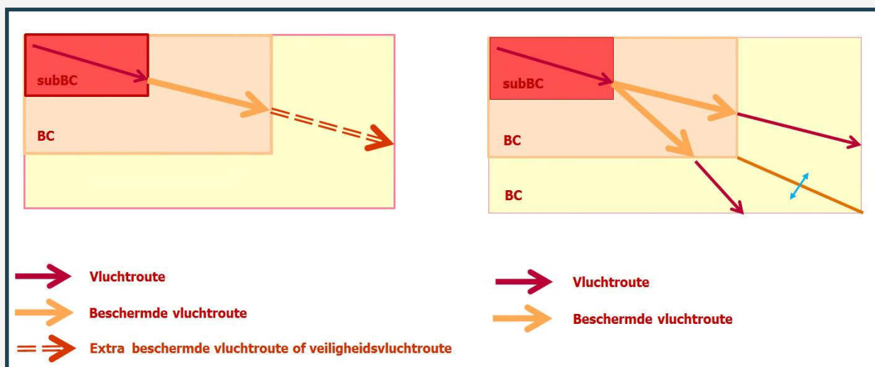
Figuur a: Ontvluchtingssystematiek bij 1 vluchtroute vanaf (bron: Ministerie BZK)
